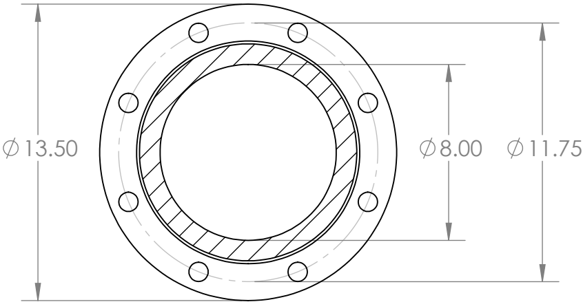
SECTION A-A SCALE 1 : 6
